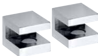
■ Držáky poliček pár Glass shelf holder - without glass, pair Halterung für Glasablagen, Paar Держатель полочки без стекла (пара) 20 x 20 x 25 mm, ≠ 8 mm 102202112
