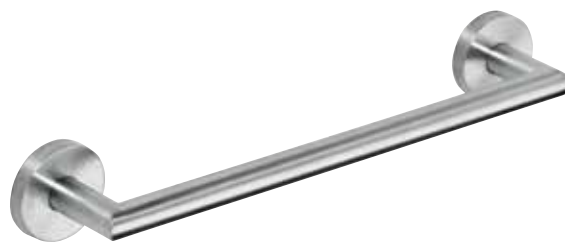
■ Držák ručníků Towel holder | Handtuchhalter Полотенцедержатель 104204015 355 x 55 x 65 mm 104204125 505 x 55 x 65 mm 104204045 655 x 55 x 65 mm
